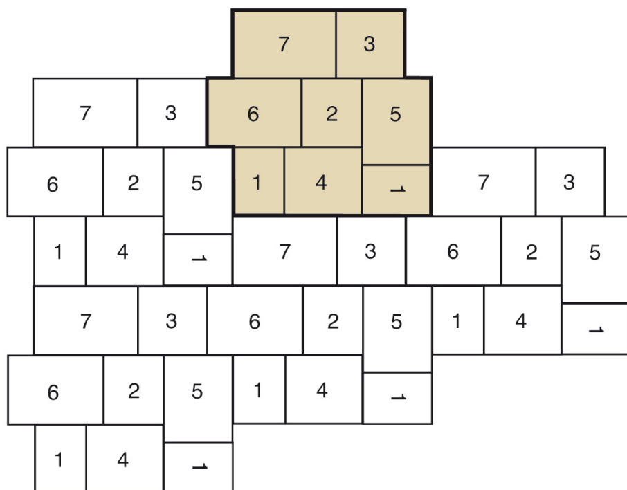
Verlegezeichnung Marktpflaster im Römischen Verband.
